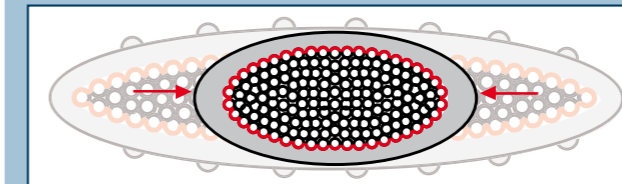
Corte transversal bajo carga (WLL) por comparación.
