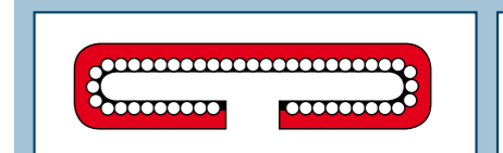
Fig.: Guaina Secutex di protezione a clip e gancio Joker
