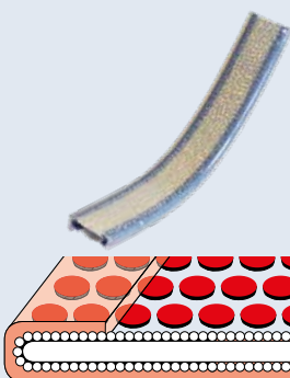
secutex®Armierung Schutz gegen tiefes Einschneiden
