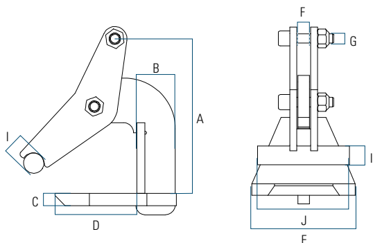
Masszeichnung zu TLH-Blechklemme
