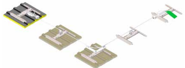
Seilsystem auf Firstbereich
