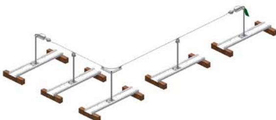
Seilsystem auf Steildach
