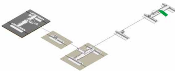
Seilsystem auf OSB/Rauschalung & Mehrschichtplatte
