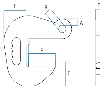
Masszeichnung zu F-Haken
