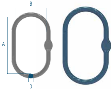
EXOSET® Öse mit Flachstelle, übergross (EN 1677)
