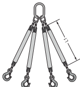
Multi-Set 4 bracci - UNI EN 1492-2 - UNI EN 1667 - C.S. 7:1
