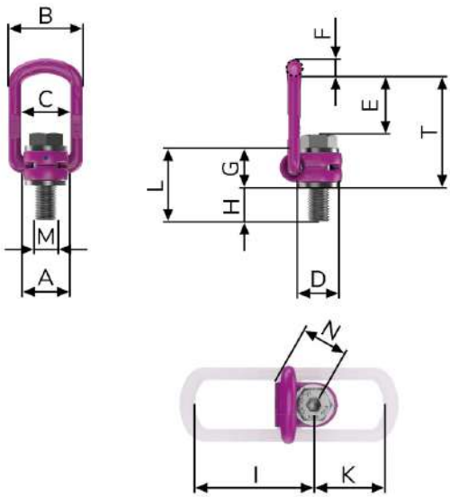
Golfari girevoli con staffa VLBG-PLUS - GR120 - EN1677 - C.S. 4:1
