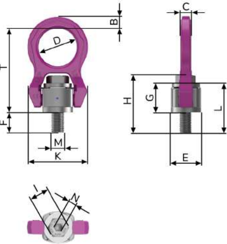
Golfari girevoli con snodo ICE ACP-TURNADO - GR120 - EN1677 - C.S. 4:1
