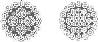
VS 16-1 - Antigiro - Lubrificazione speciale - Cod. FyVS16100-rrr
