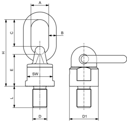
Golfare girevole con anello - GR100 - EN1677 - C.S. 4:1
