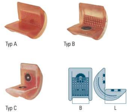
Paraspigolo a 90° - SWH Tipo A: senza calamita Tipo B: con calamita inferiore Tipo C: con calamita su entrambi i lati
