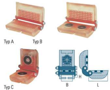
Paraspigolo con snodo - SK-B Tipo A: senza calamita Tipo B: con calamita inferiore Tipo C: con calamita su entrambi i lati
