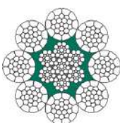
VS 8-7CP - Compattata - Plastificata - Lubrificazione speciale - Cod. FyVS8700CP-rrr
