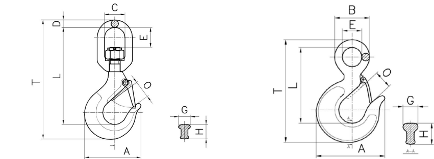
Gancio girevole al carbonio C.S. 5:1 - Acciaio legato C.S. 4:1
