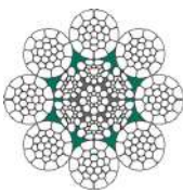
VS 8-2CP - Compattata - Plastificata - Lubrificazione speciale - Cod. FyVS8200CP-rrr
