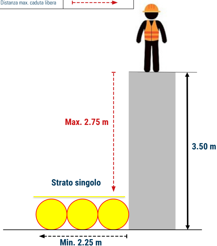
Grafico altezza massima per installazione a strato singolo
