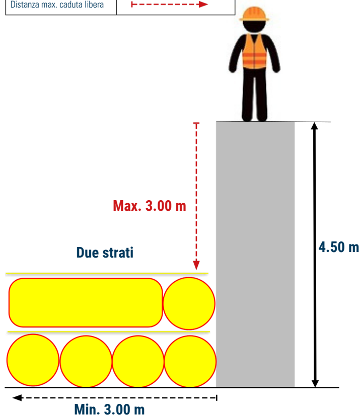
Grafico altezza massima per installazione a due strati
