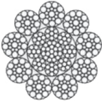
9x19 IWRC Excellent Bend Fatigue values
