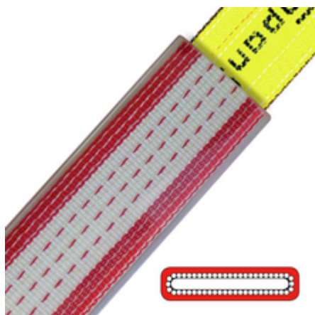
Secutex - SF2 Nastri piatti con doppio rivestimento
